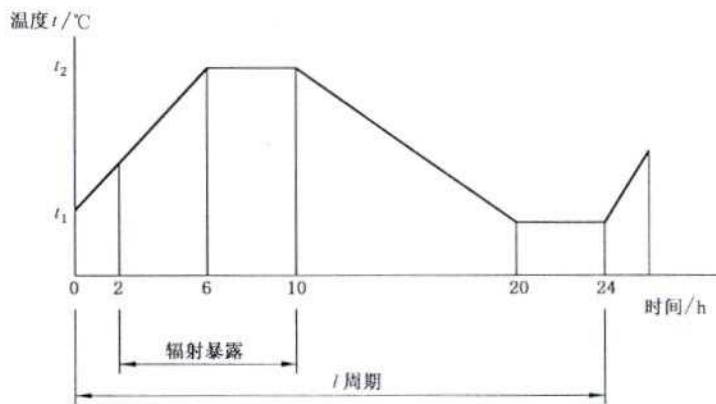
图 1 适用于严酷等级 01 的可控试验箱(室)温度和辐射暴露周期的试验程序(所需的三个周期之一)
