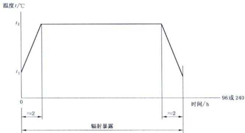
图3 适用于严酷等级03和04的可控试验箱(室)温度和辐射暴露周期的试验程序
