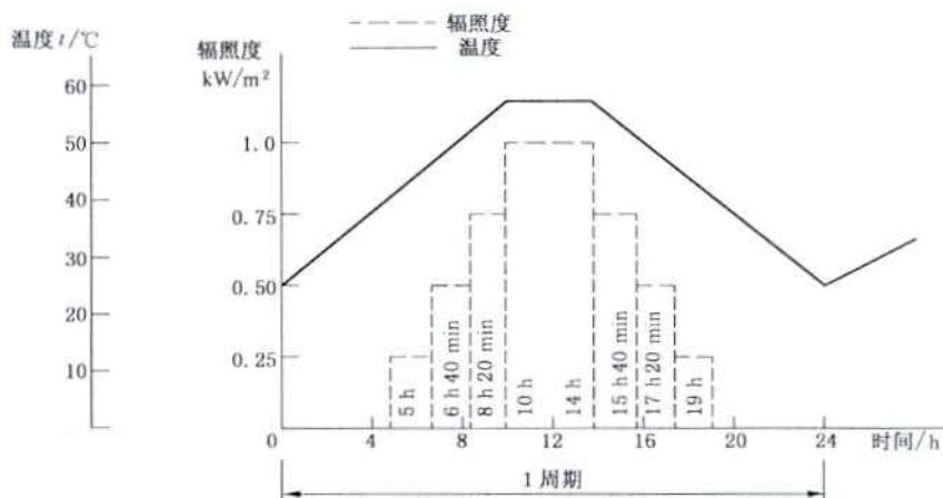
图 2 适用于严酷等级 02 的辐照度和可控试验箱(室)温度的试验程序(所需的五个周期之一)
